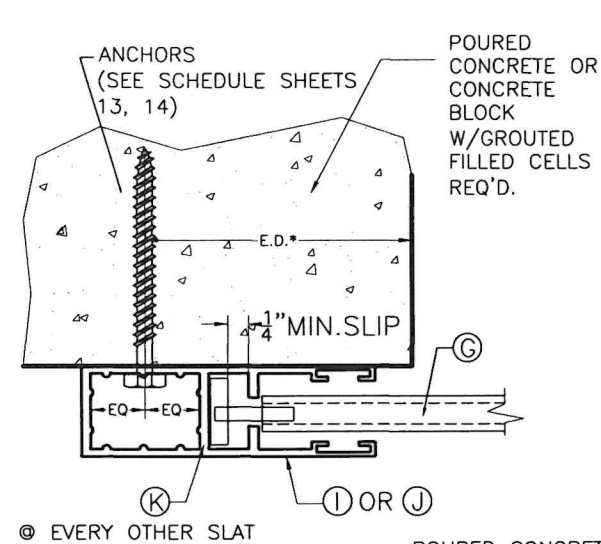
SECTION J-J : WALL MOUNT
